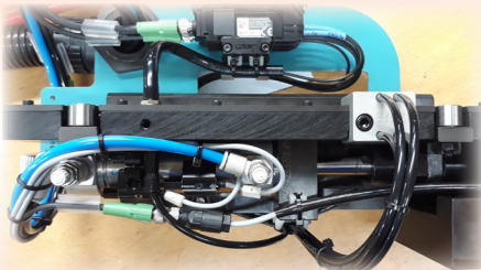
Cassette supérieure avec poinçons de formage et découpe
