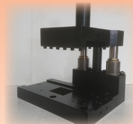
INTERFACE POUR MONTAGE SUR PRESSE D'AUTRE MARQUE QUE SEREC
