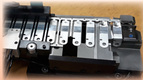
Embase porte matrices de découpe et formage pliage
