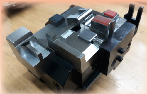
Cassette supérieure avec poinçons de formage et découpe
