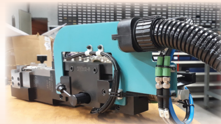
Raccordements électriques et pneumatiques
